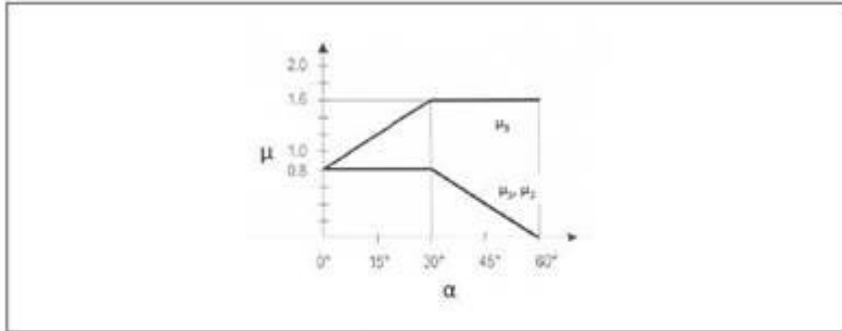
Kuva 5.1S. Lumikuorman muotokertoimet.
